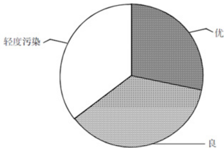
图2 上海2015年3月空气质量分布情况
