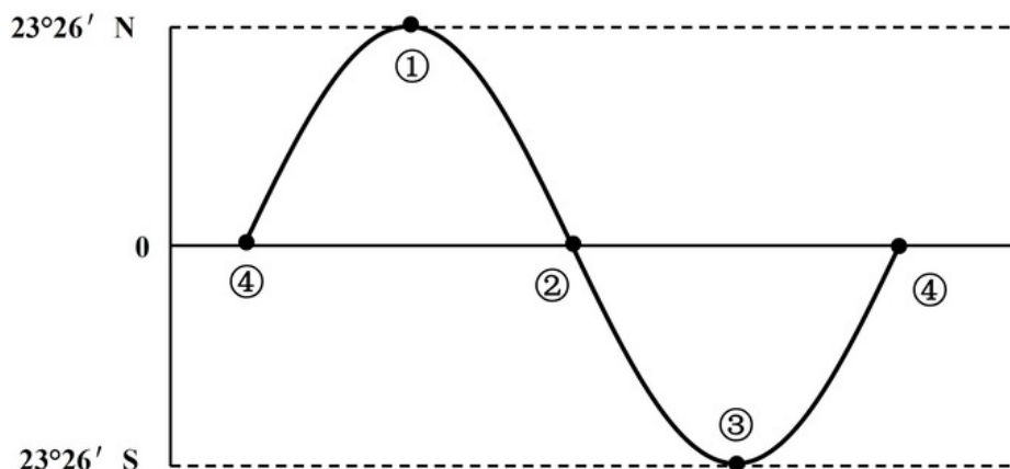
太阳直射点移动图
